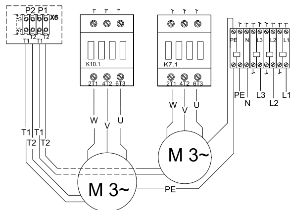
Рис. 29 Схема соединений для Multilift MD/MLD.22.3.4 с трехфазным электродвигателем с контакторами
