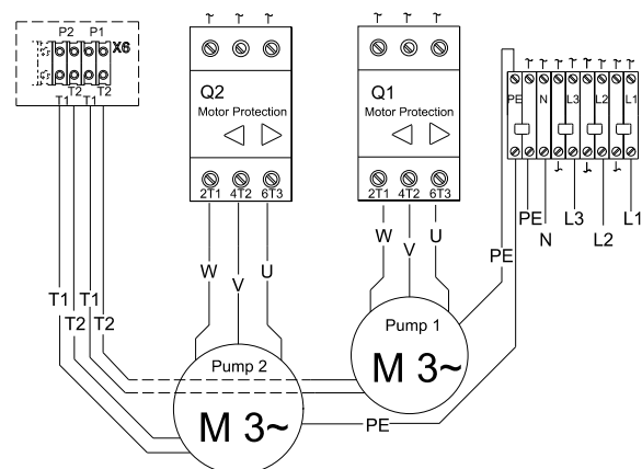
Рис. 30 Схема соединений для Multilift MD/MLD.24.3.2, MD/MLD.32.3.2 и MD/MLD.38.3.2 с трехфазным электродвигателем с дополнительным автоматом защитного отключения
