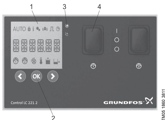
Рис. 9 Панель управления
