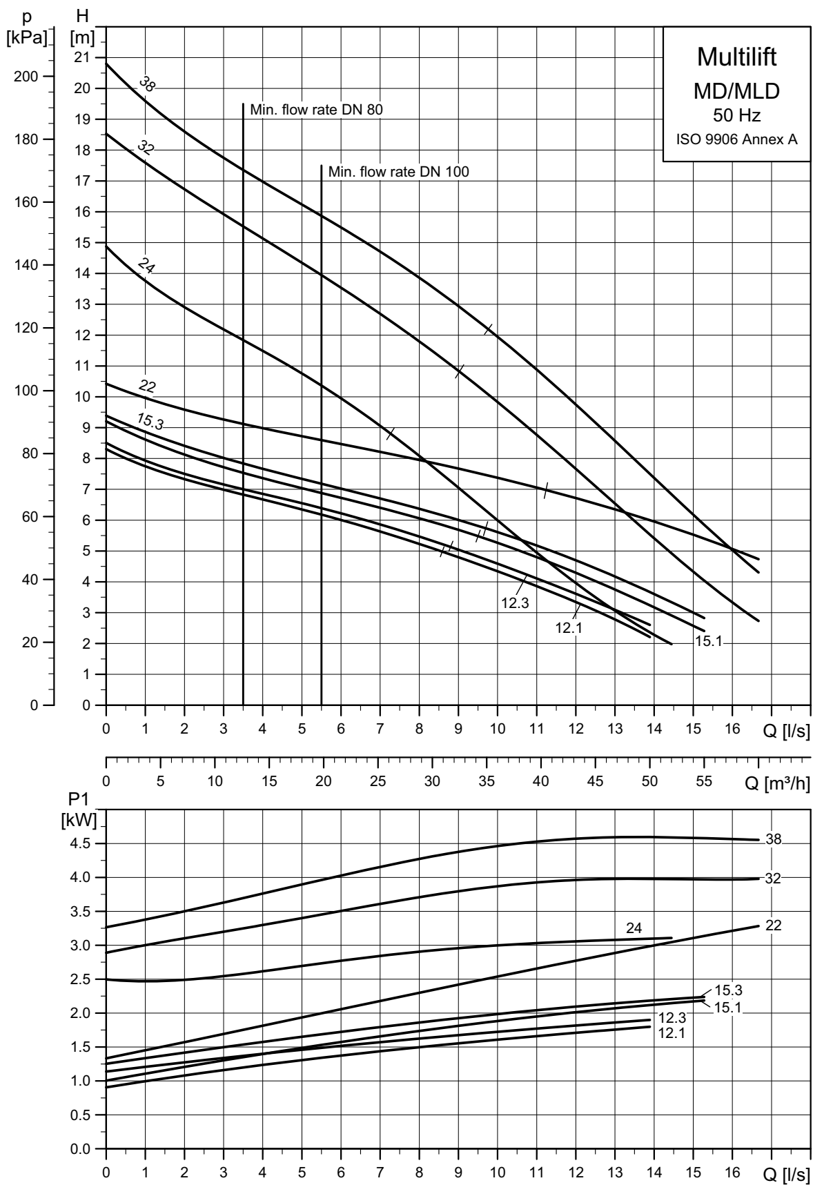
Рис. 36 Рабочие характеристики
